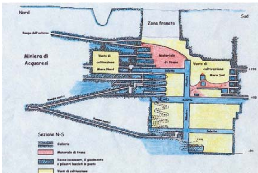
Fig 2 - Schema di coltivazione e dei crolli 1991-1998
