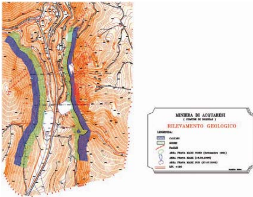
Fig. 4 - Geologia dell'area di Acquaresi
